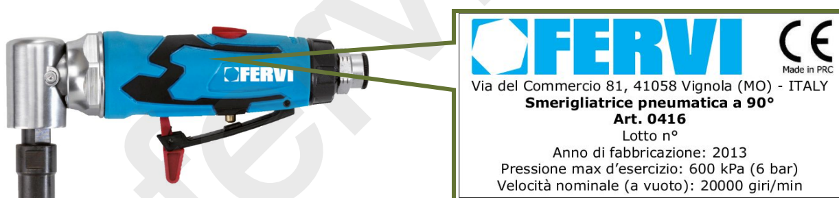
Figura 3 – Dettaglio targhetta di identificazione
