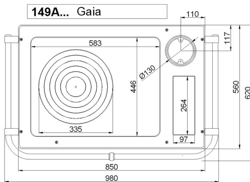
Medidas en mm de los modelos de equipo
