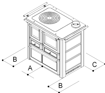
Medidas en mm de los modelos de equipo
