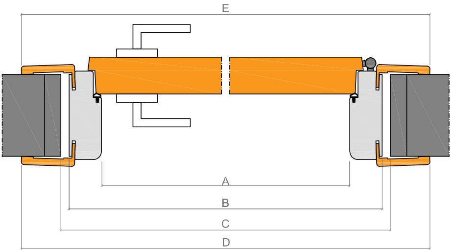
SEZIONE ORIZZONTALE
