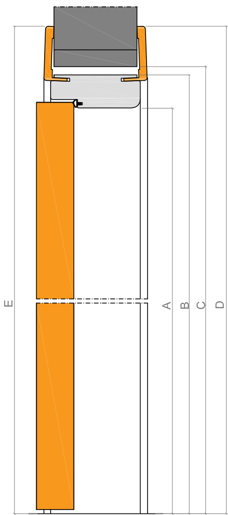
SEZIONE VERTICALE
